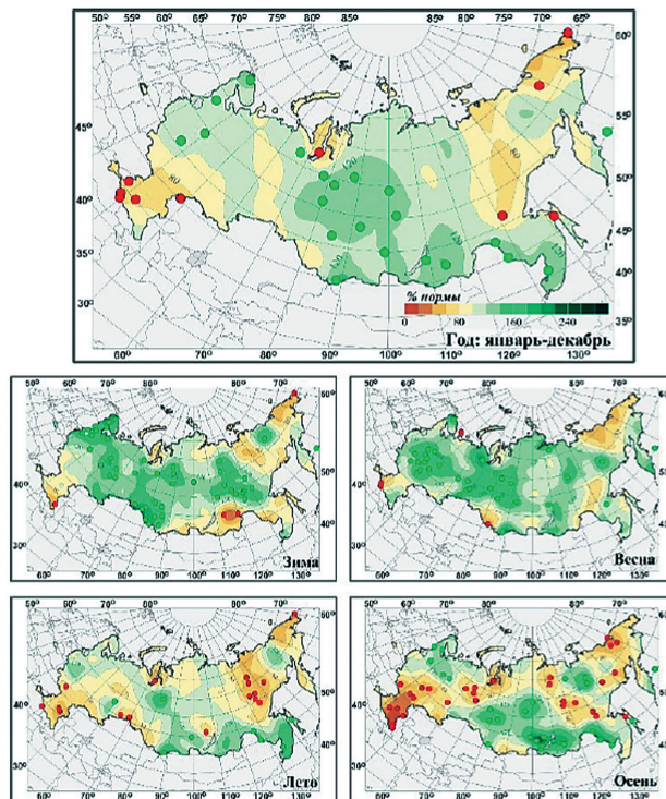
Рисунок 3.6 – Аномалии осадков на территории Российской Федерации в 2020 г., с указанием локализации 5%-х экстремумов (красные кружки) и 95%-х (зеленые кружки) Источник: Доклад об особенностях климата на территории Российской Федерации за 2020 г. Росгидромет, 2021
