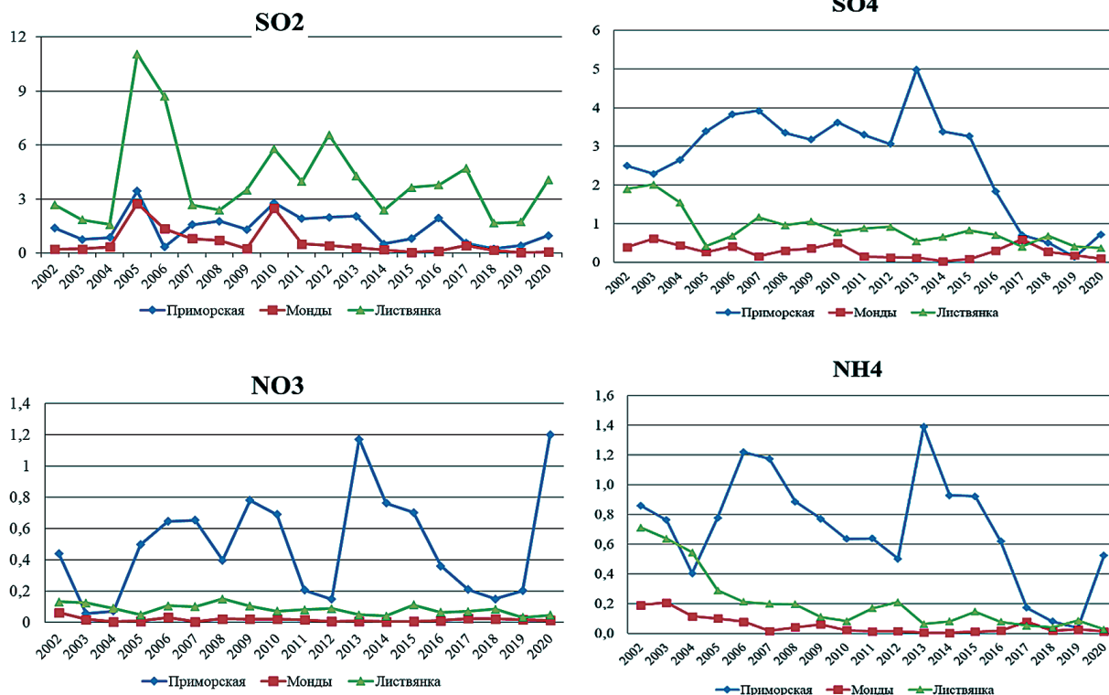
Рисунок 2.12 – Изменения средних годовых концентраций соединений серы (сверху) и азота (снизу) в воздухе на станциях ЕАНЕТ (мкг/м³)
