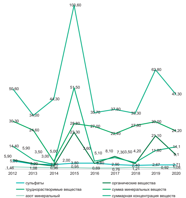
Рисунок 13.1 — Динамика поступления химических веществ из атмосферы на ст. Хамар-Дабан, тонн/год на км 2
