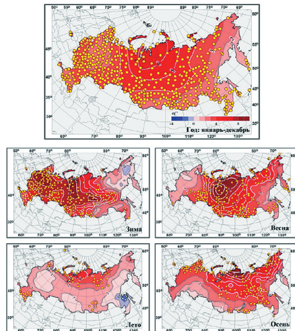
Рисунок 3.2 – Аномалии средней годовой и сезонных температур приземного воздуха на территории Российской Федерации в 2020 г. (отклонения от средних за 1961–1990 гг.) с указанием локализации 95%-х экстремумов (желтые кружки)
